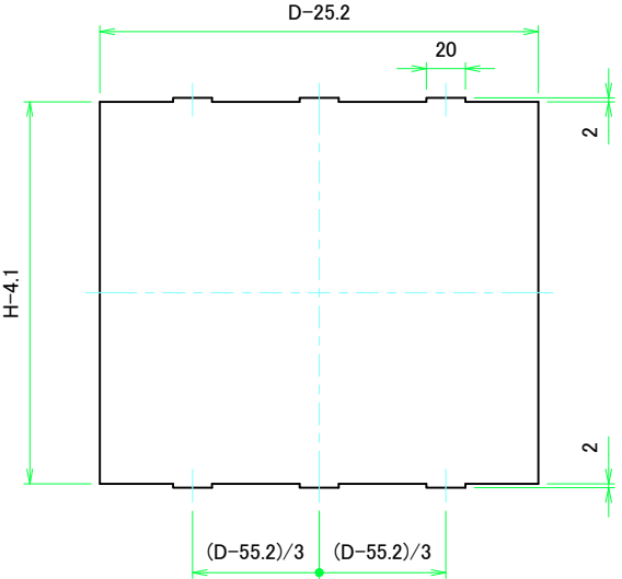
Dパネル1表面 / D Panel 1 Frontside
