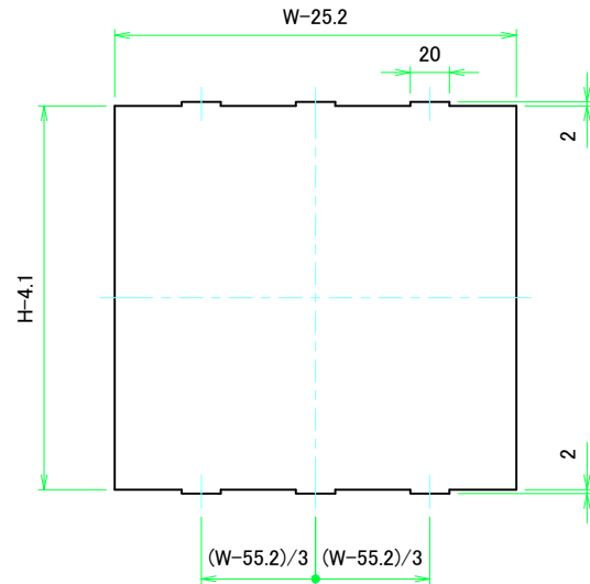
Wパネル1表面 / W Panel 1 Frontside
