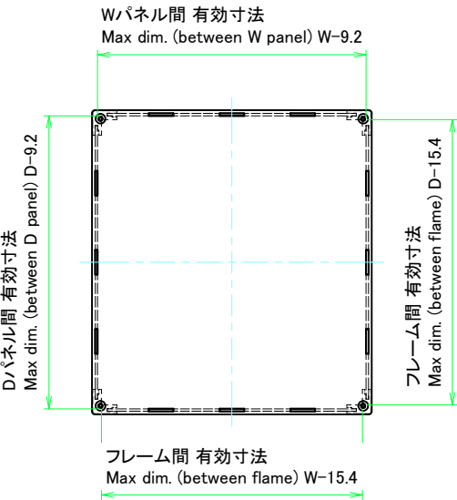
下カバー / Bottom cover
